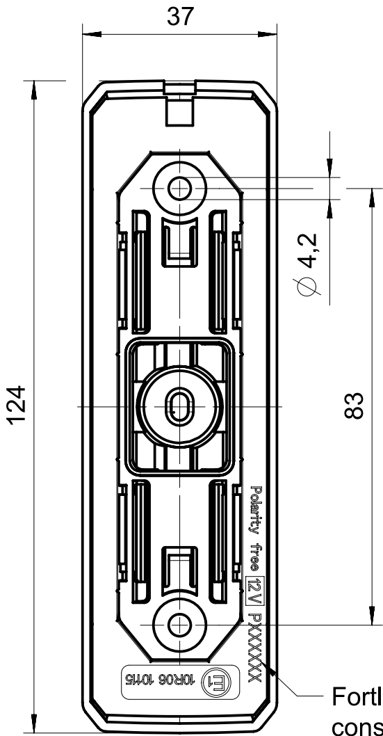
Ansicht ohne Kabel / view without cable
